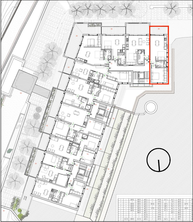
Unità 5A - Piano Primo
